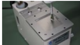
BGA リポールツール
